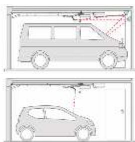
Laser & reflektor
